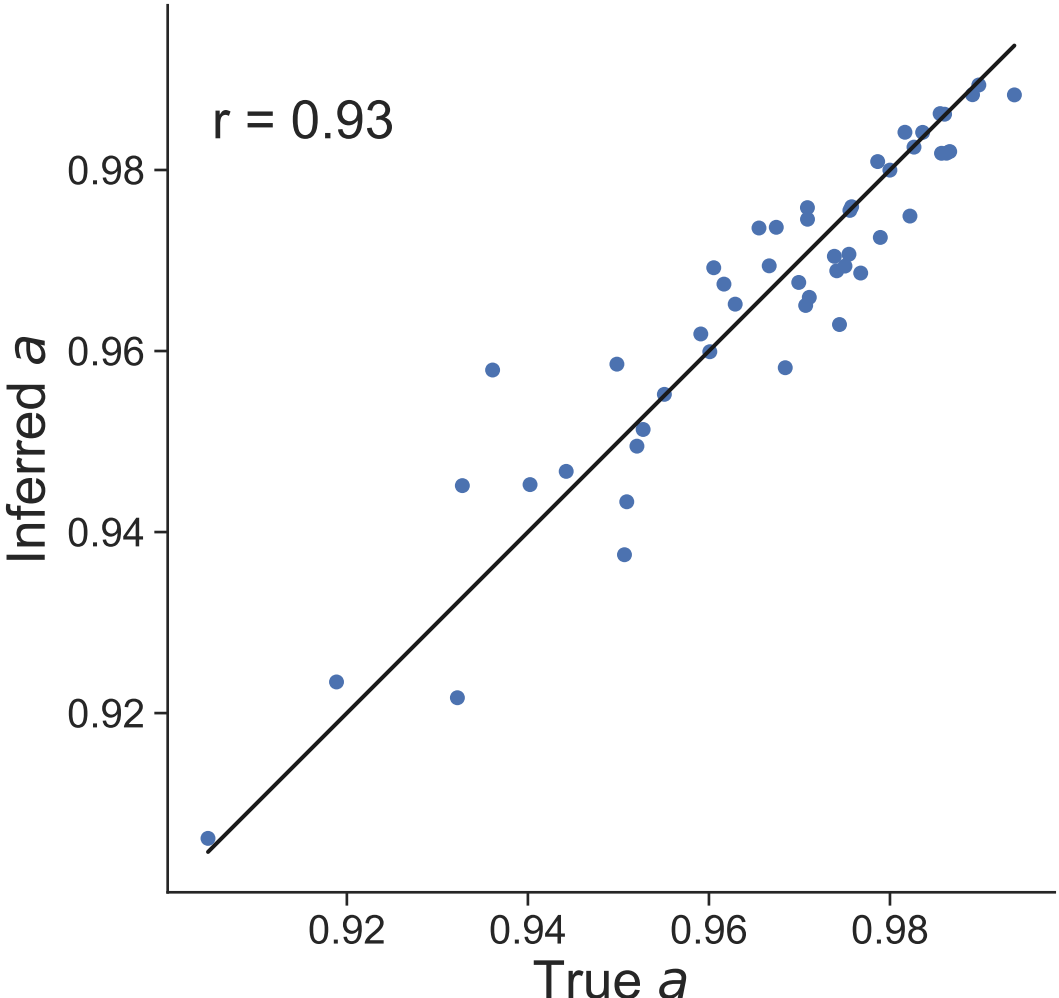
Dataset 24
