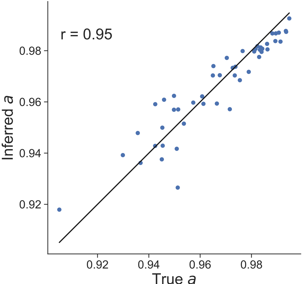
Dataset 5
