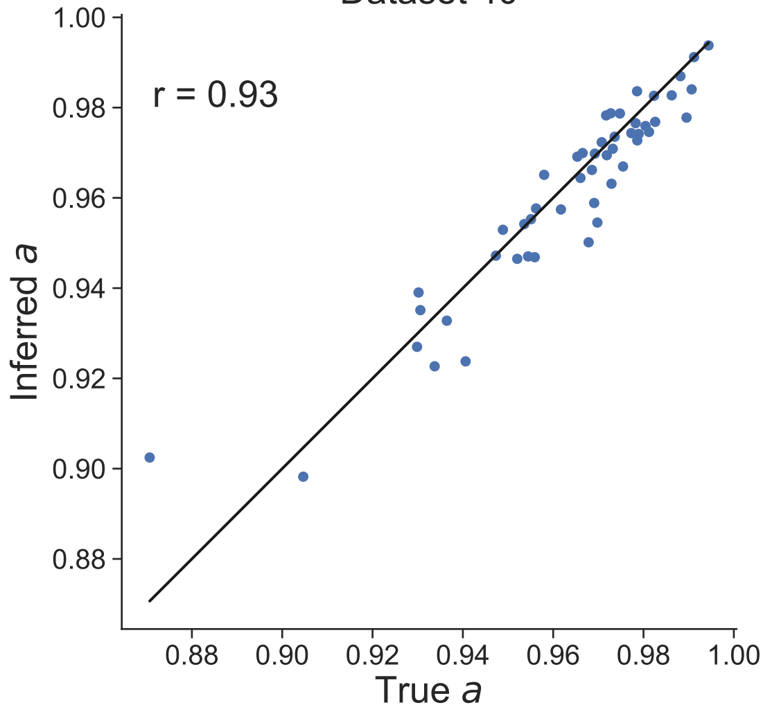
Dataset 40
