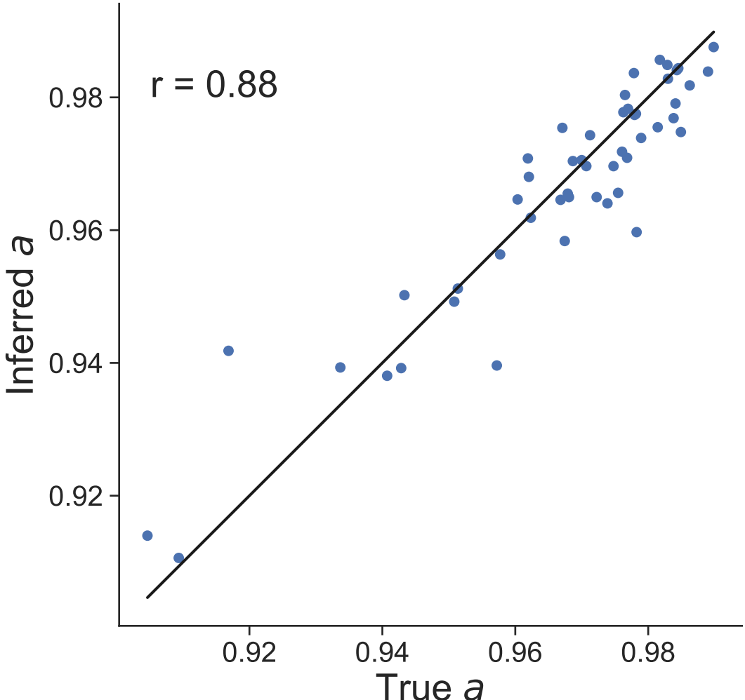
Dataset 11
